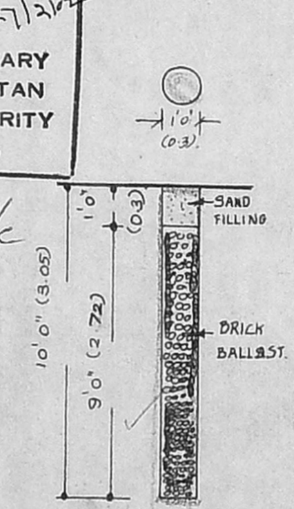
PERCOLATION PIT.
