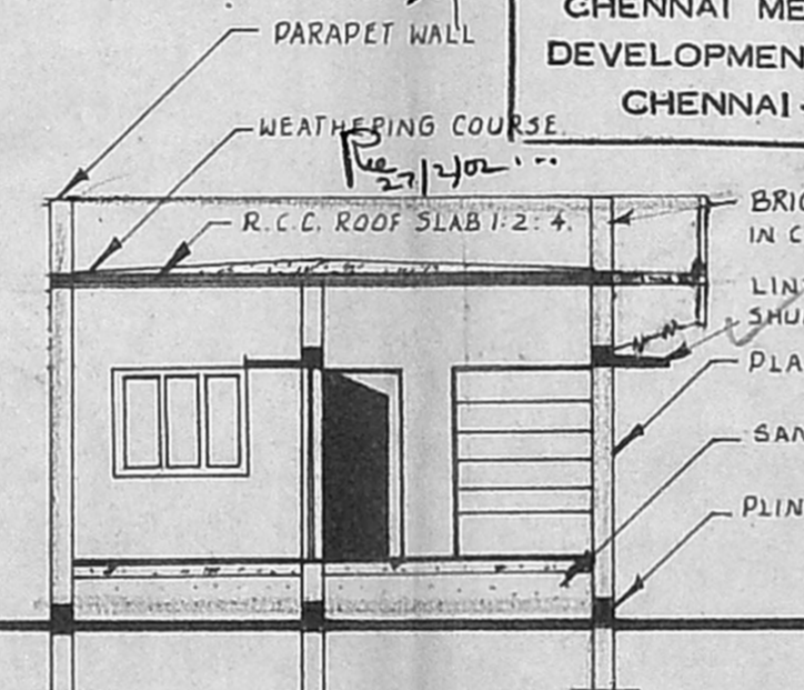
SECTION ONA-B
